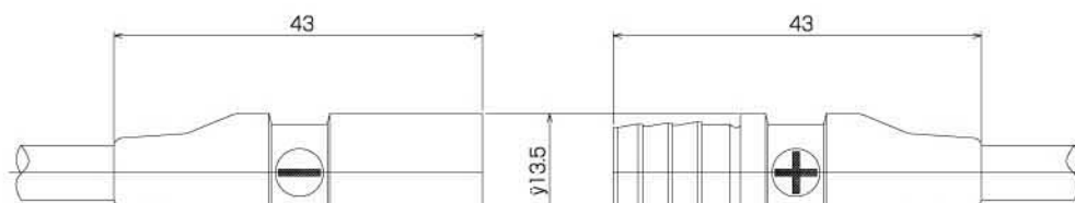
メス側組立品番(KTN-PVC1P-F)
