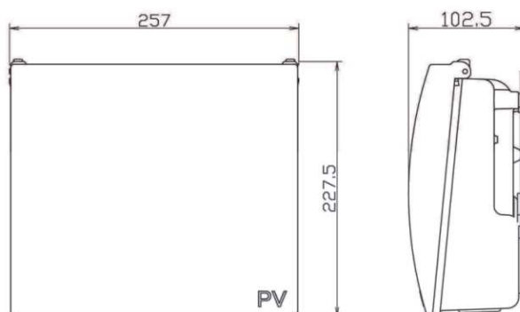
<製品寸法図>
