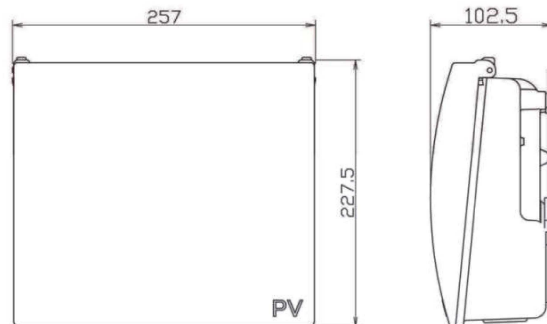
<製品寸法図>
